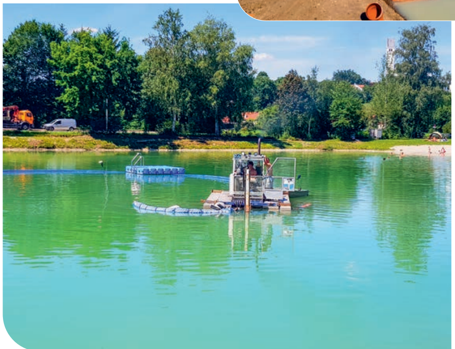
Das schwimmende Steuerfahrzeug, mit dem der Unterwasserroboter gelenkt wurde.
