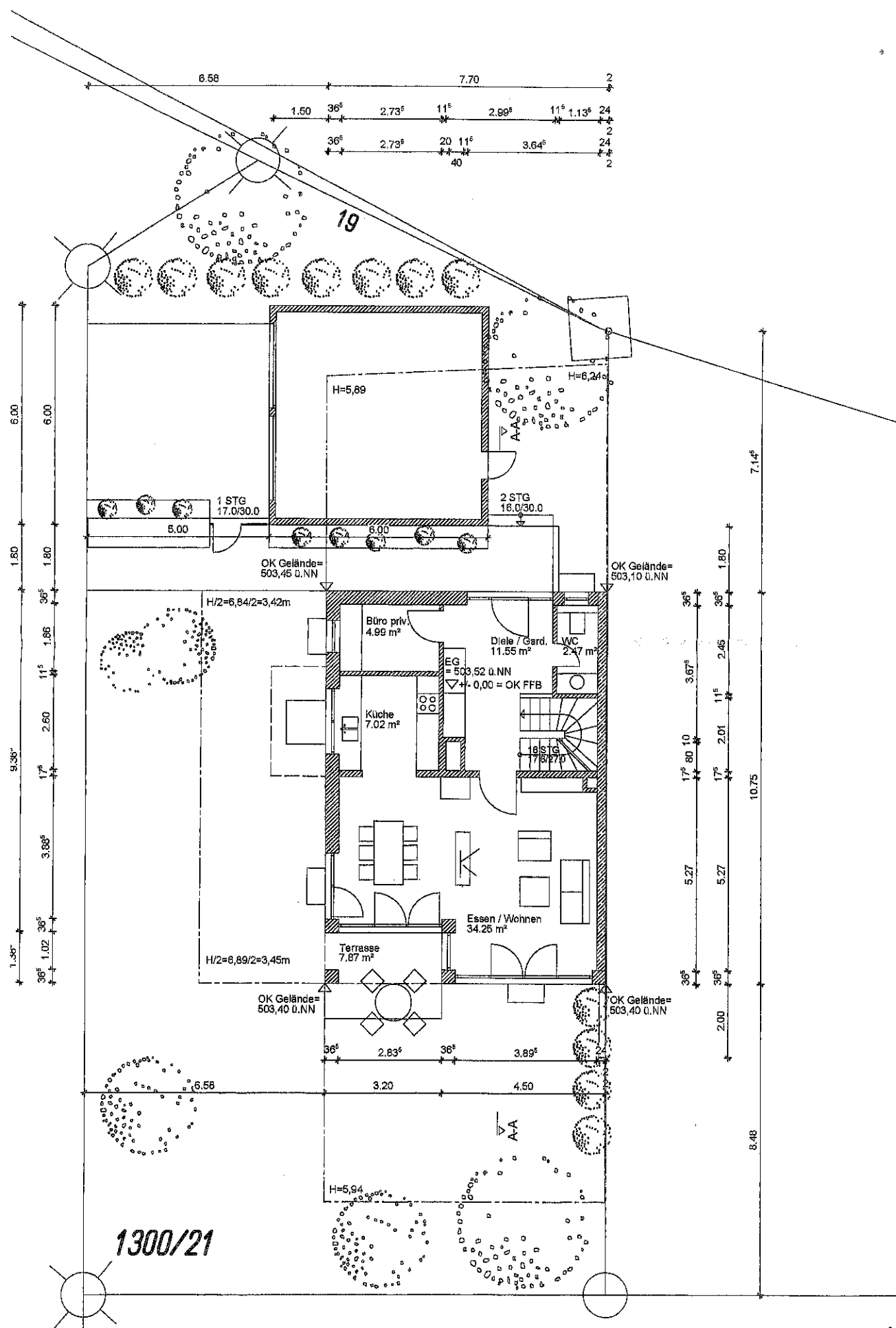
Grundriss Erdgeschoss
